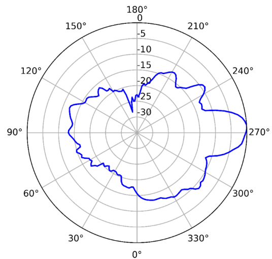
2.4GHz (Vertical)
