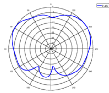
2.4G (Vertical)
