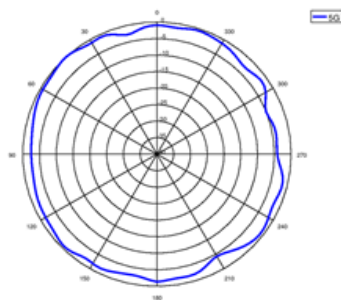
5G (Horizontal)
