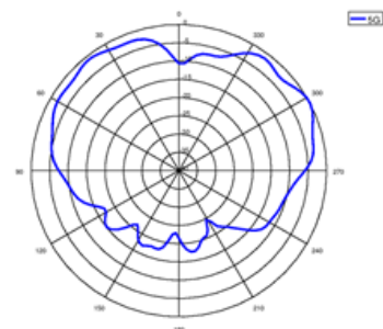
5G (Vertical)
